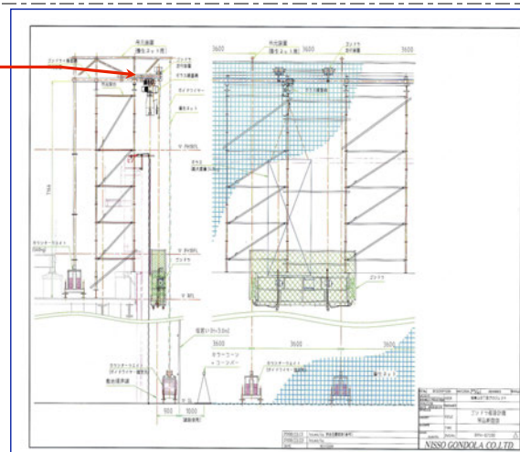
《吊元断面図》
