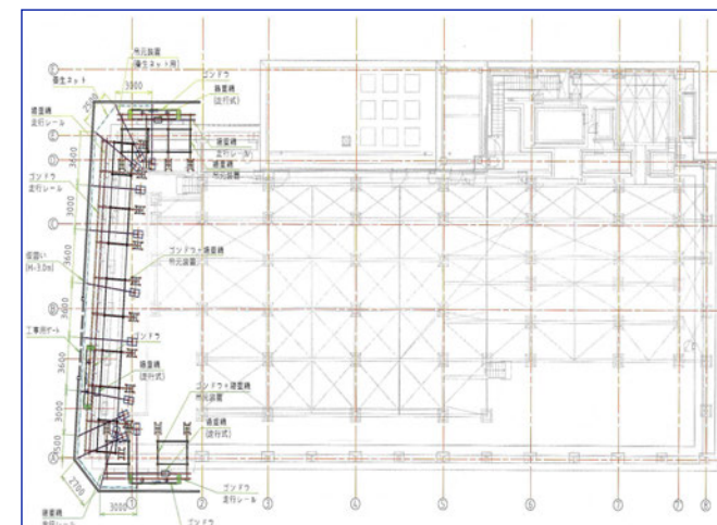
《全体平面図》
