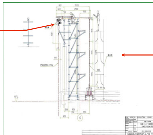
《吊元断面図》
