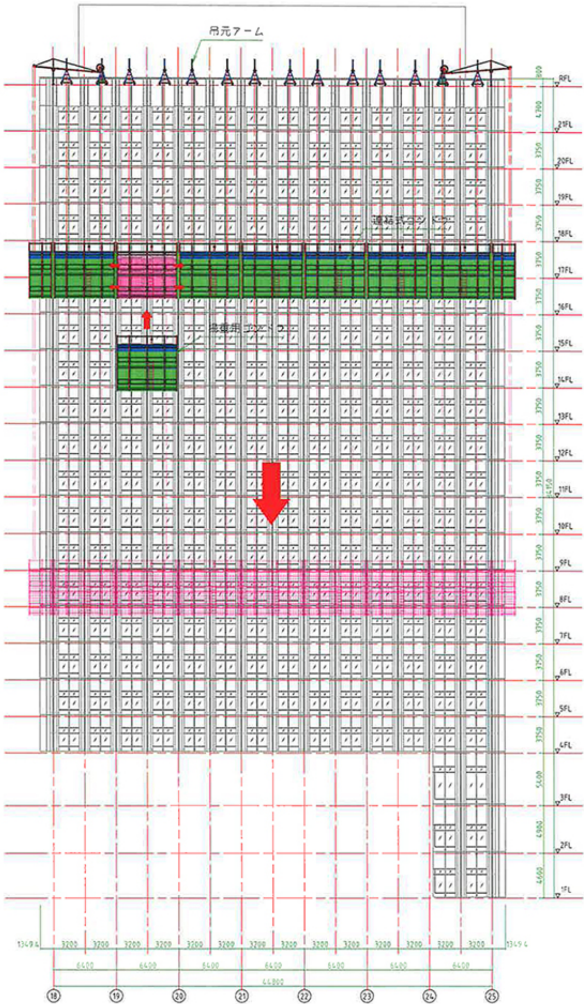
南立面图
