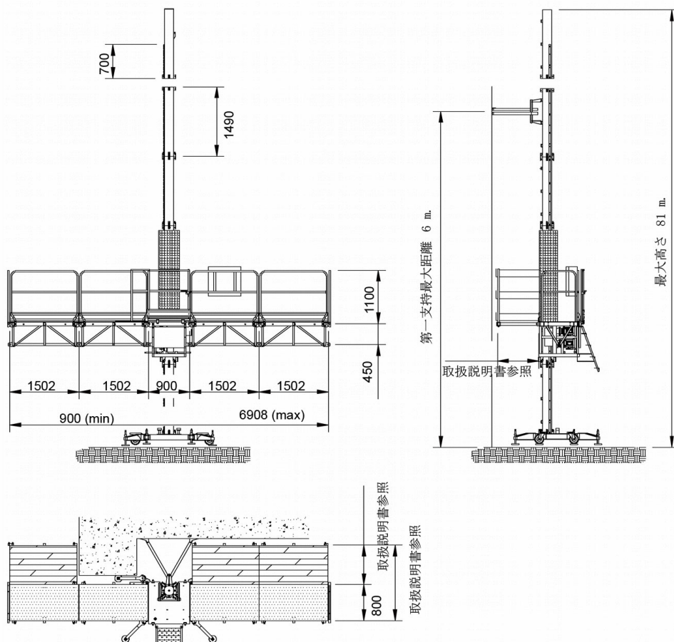
シングルマストワークプラットフォーム ELSA P25/7 SINGLE MAST CLIMBING WORK PLATFORM ELSA P25/7
