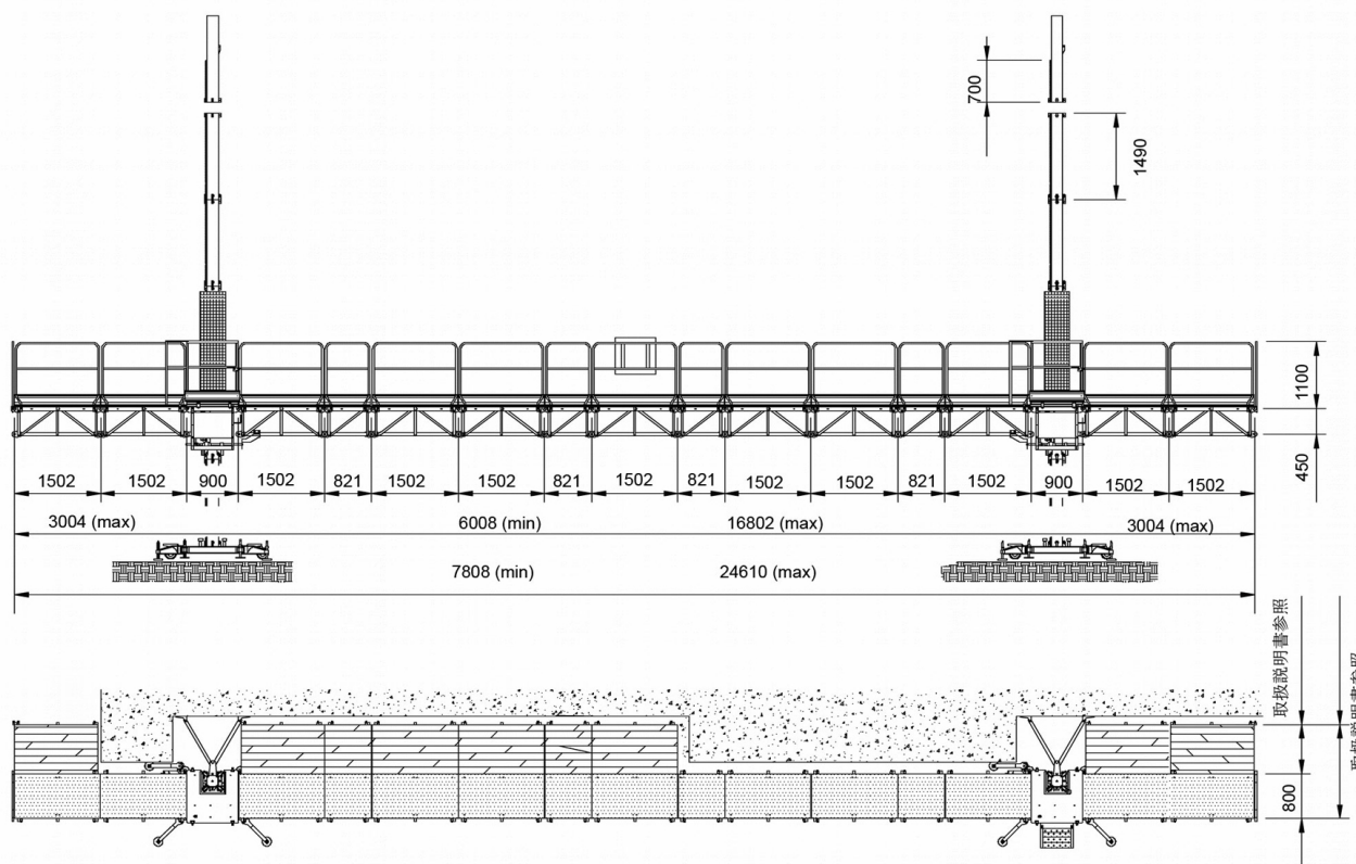
ツインマストワークプラットフォーム ELSA P25/25 TWIN MAST CLIMBING WORK PLATFORM ELSA P25/25
