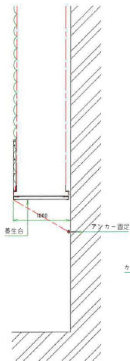
養生台 + アンカー
