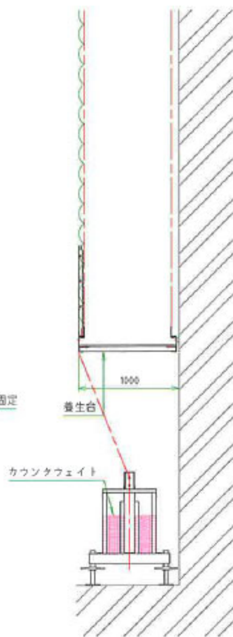
養生台 + カウンタウェイト
